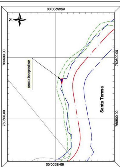
PLANO DE UBICACIÓN Esc. 1:2.000
